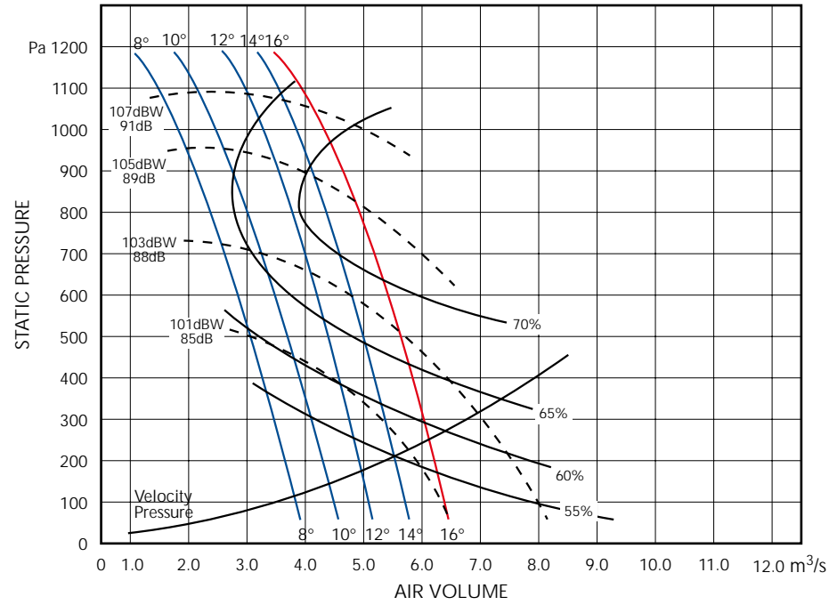
LC63A2 / 3ph
