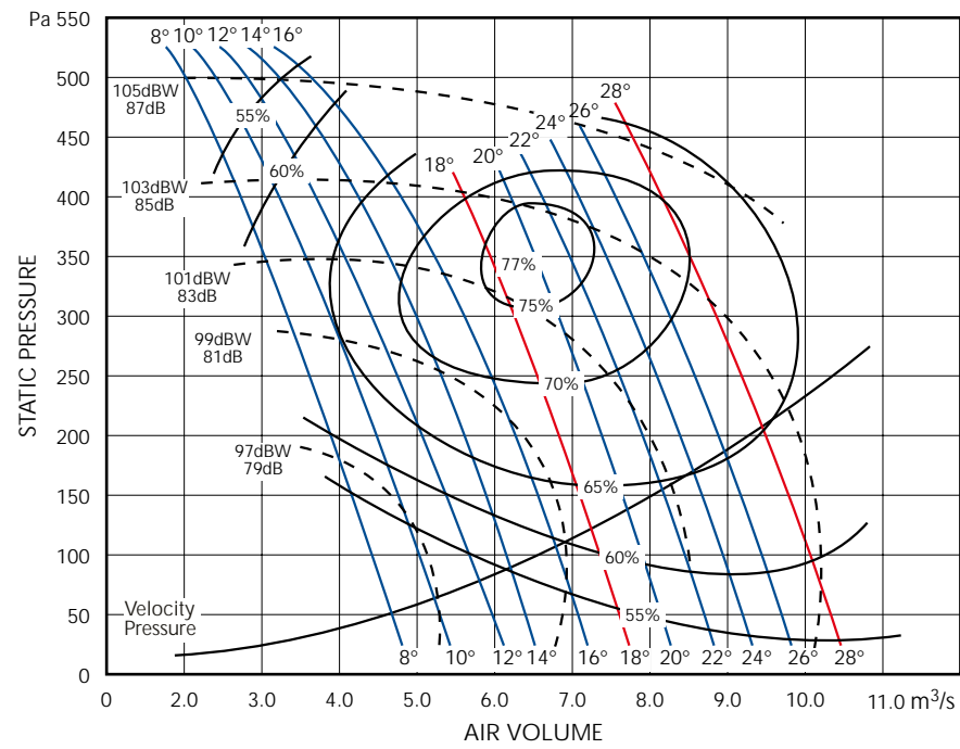
LC80A4 / 3ph
